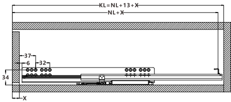
内置抽屉 Inner Drawer
